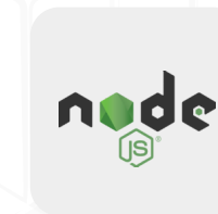
NodeJS
