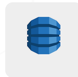
Amazon DynamoDB
